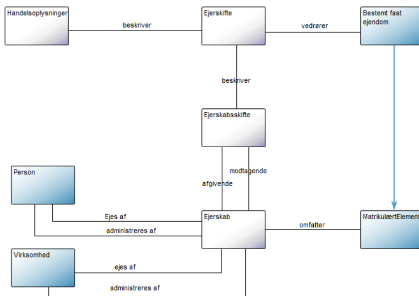
Figur 1- Objektmodel for byggeblok Ejerskab
